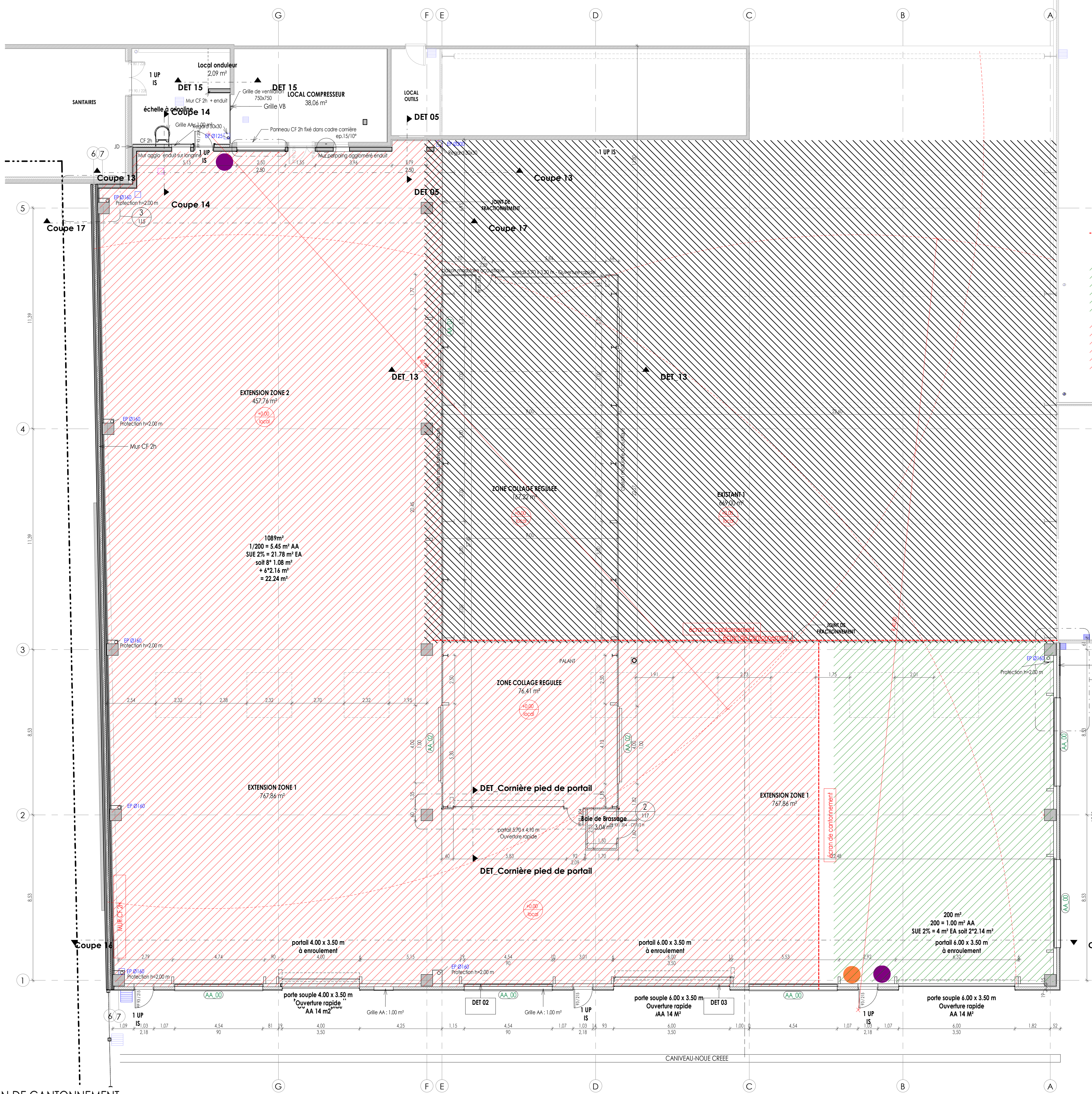
PLAN DE CANTONNEMENT Echelle : 1 : 100
